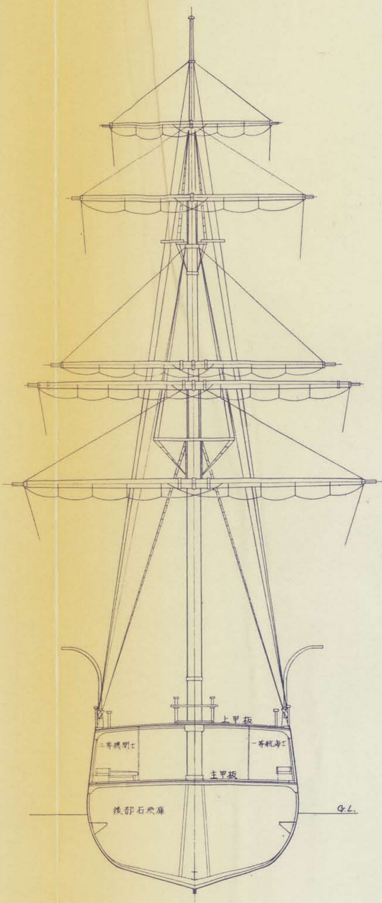
メインマスト横断面図
