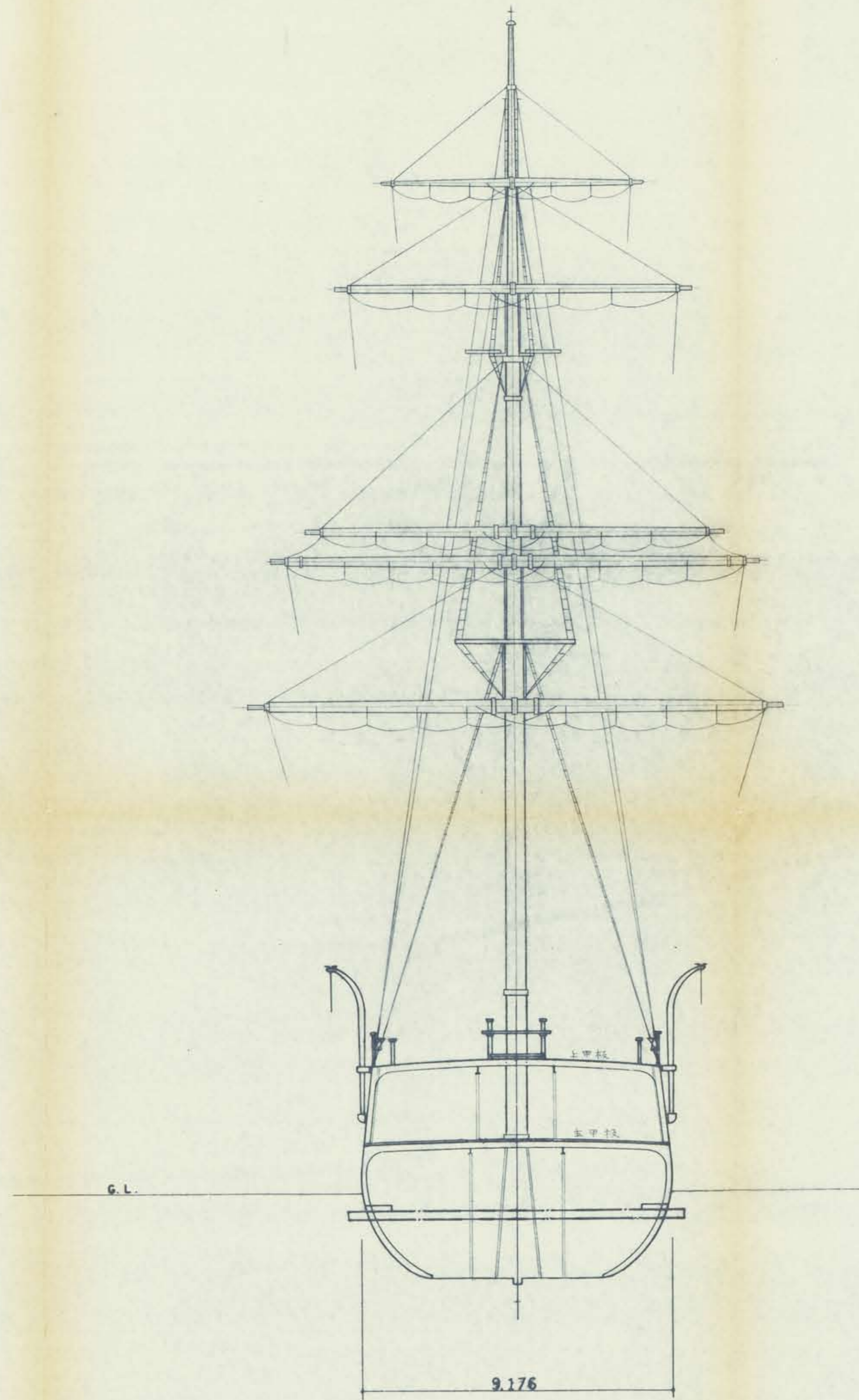
メインマスト横断面図
