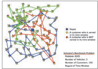
時間枠付き配送計画問題
