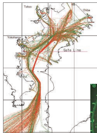
レーダによる船舶動静の計測
