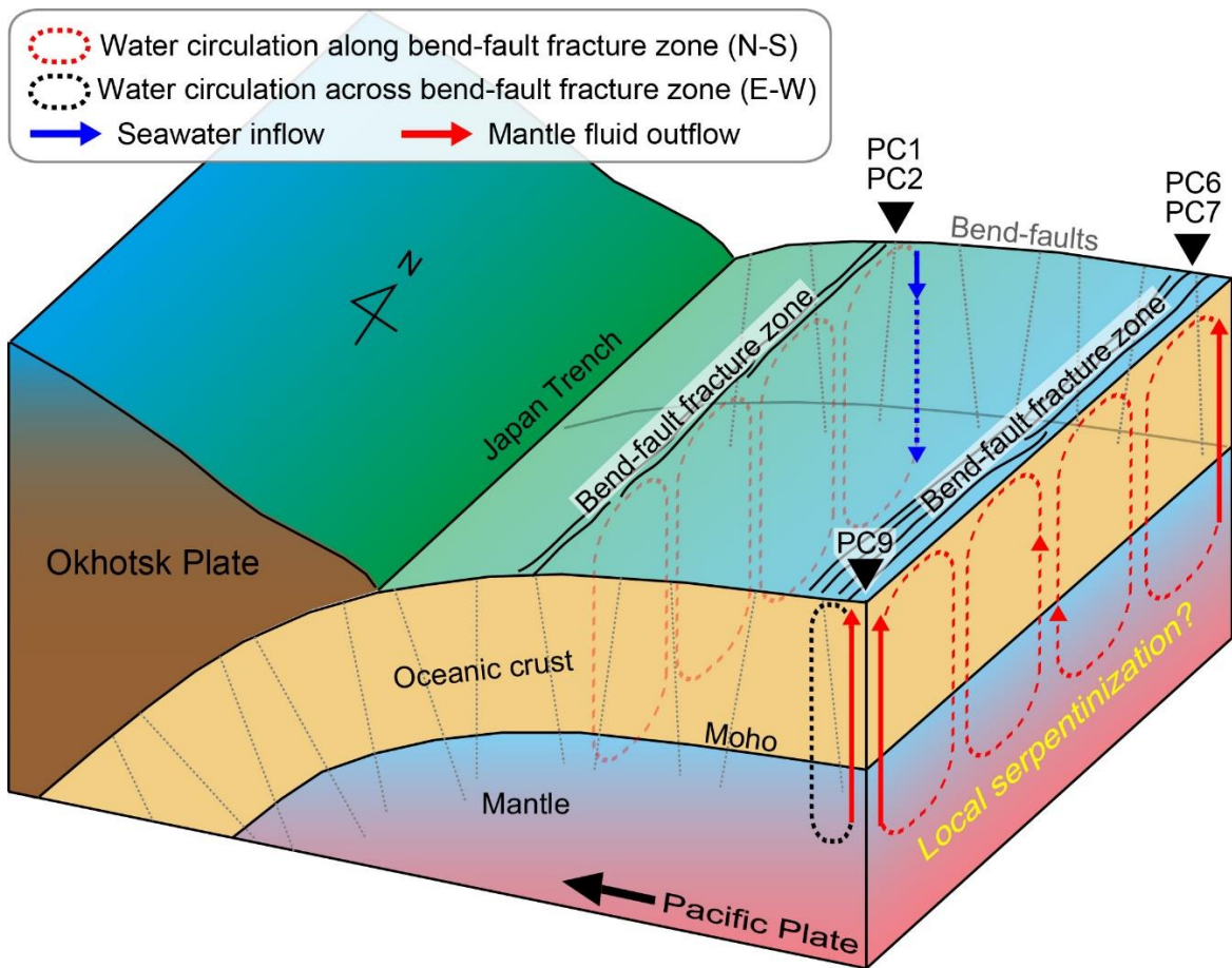
図4. 東北沖日本海溝のアウトアーライズにおける流体循環モデル。海洋プレートの屈曲による正断層（灰色点線）、マントルと海洋を結ぶ流体循環（赤点線と黒点線の長方楕円）。
