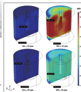
コンピューターシミュレーションによる殺菌価分布の予測
