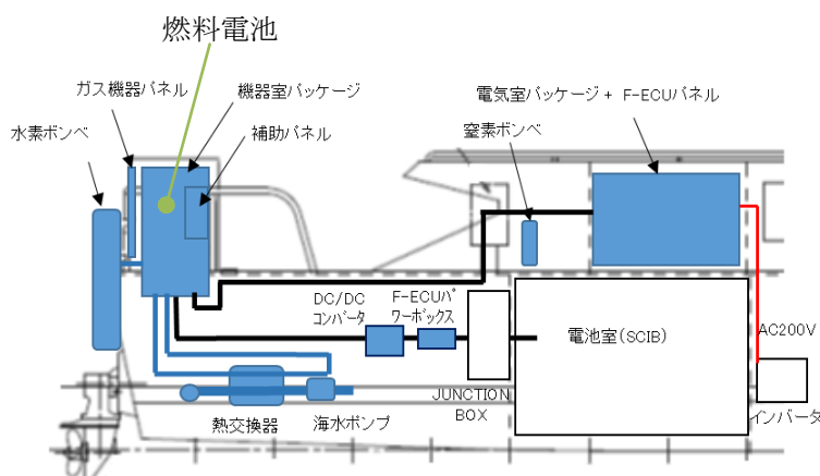
燃料電池を搭載した「らいちょう N」
